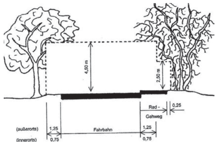
Lichtraumprofil nach § 28, Absatz 2
