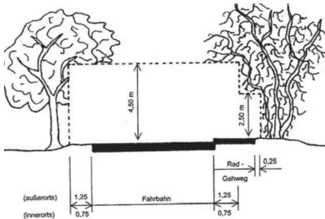
Lichtraumprofil nach § 28, Absatz 2
